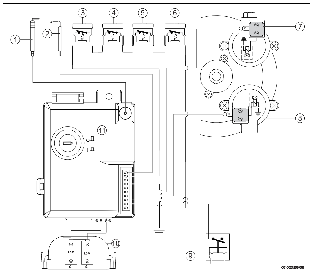
Fig. 31 Esquema elétrico
